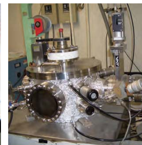
▲マグネトロンスパッタ装置
